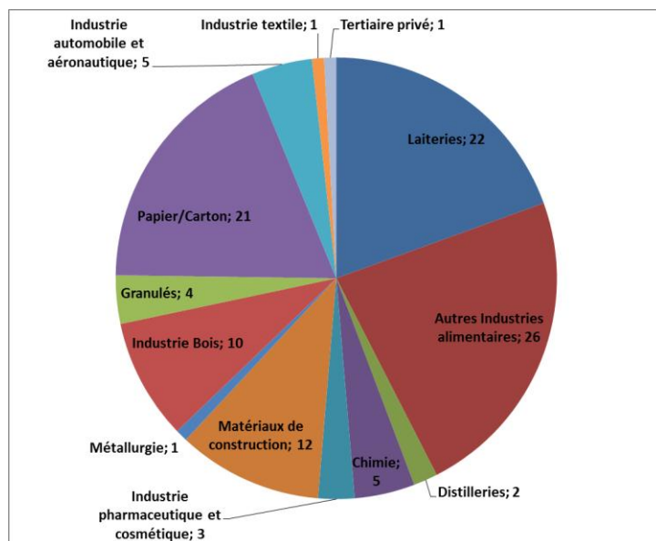
Nombre d'installations BCIAT par secteur d'activité (de 2009 à 2014) réalisées ou en cours
